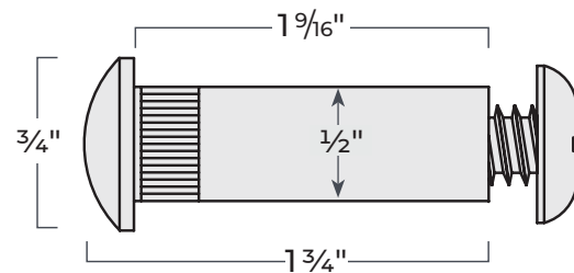
FDTB 1/2"
