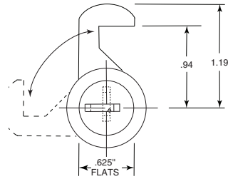
3706-144 (Coin Box)
