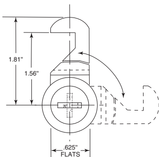
3500-100 (Door)
