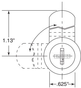
330-148 (Old Door Knob Latch)
