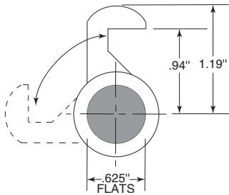
3500-100 (Door)
